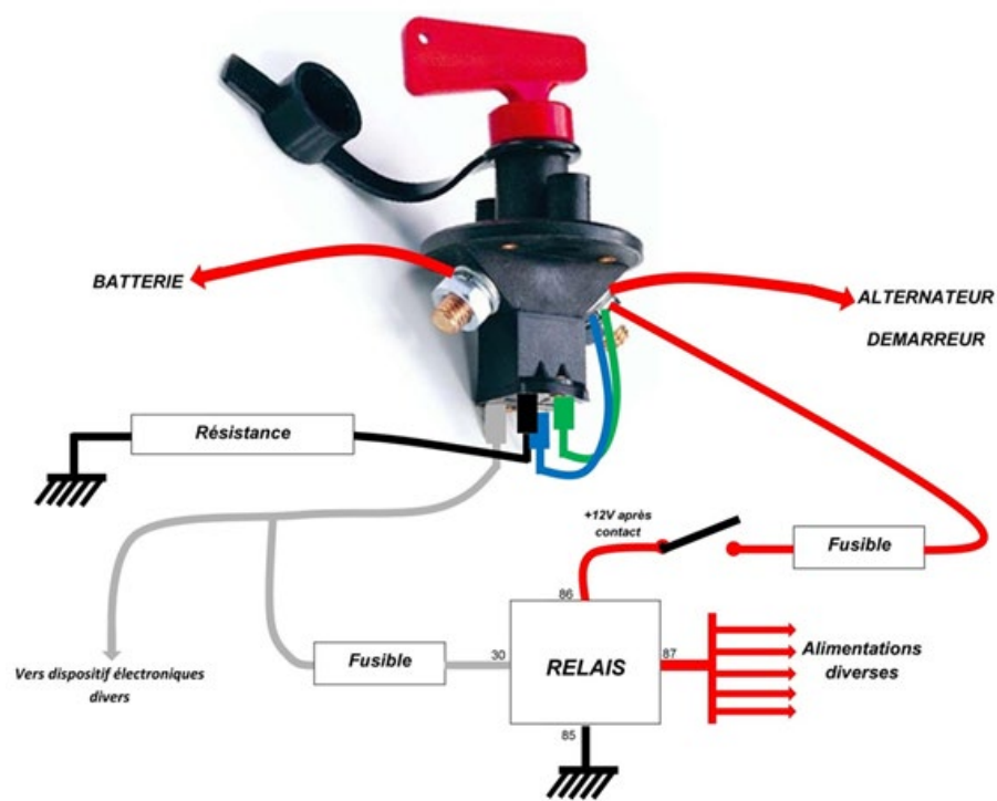
Schéma de principe COUPE-CIRCUIT
